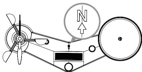
Noordelijke markering bovenop de 7-in-1 sensor.
